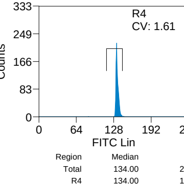
Cyan_FlowCheck_10_Sep_12 (G...
