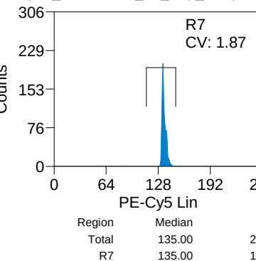
Cyan_FlowCheck_10_Sep_12 (G...
